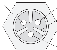
Vue A-A
