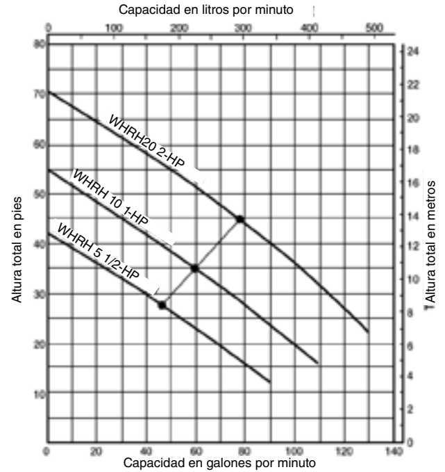
Curva de rendimiento Bombas para el manejo de desechos de la serie WHRH
