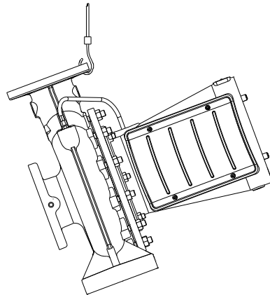
Elevación correcta de una bomba sin motor
