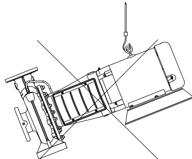
Elevación incorrecta de una bomba
