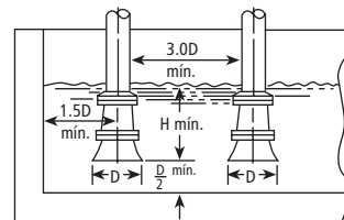
Figura 4 Tubería - Descarga
