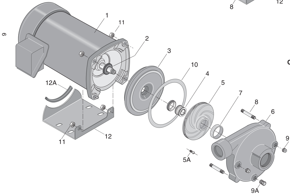
Stud Configuration
