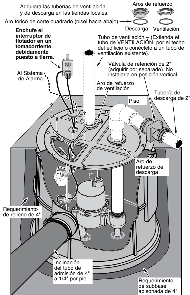
Figura 1 – Instalación típica
