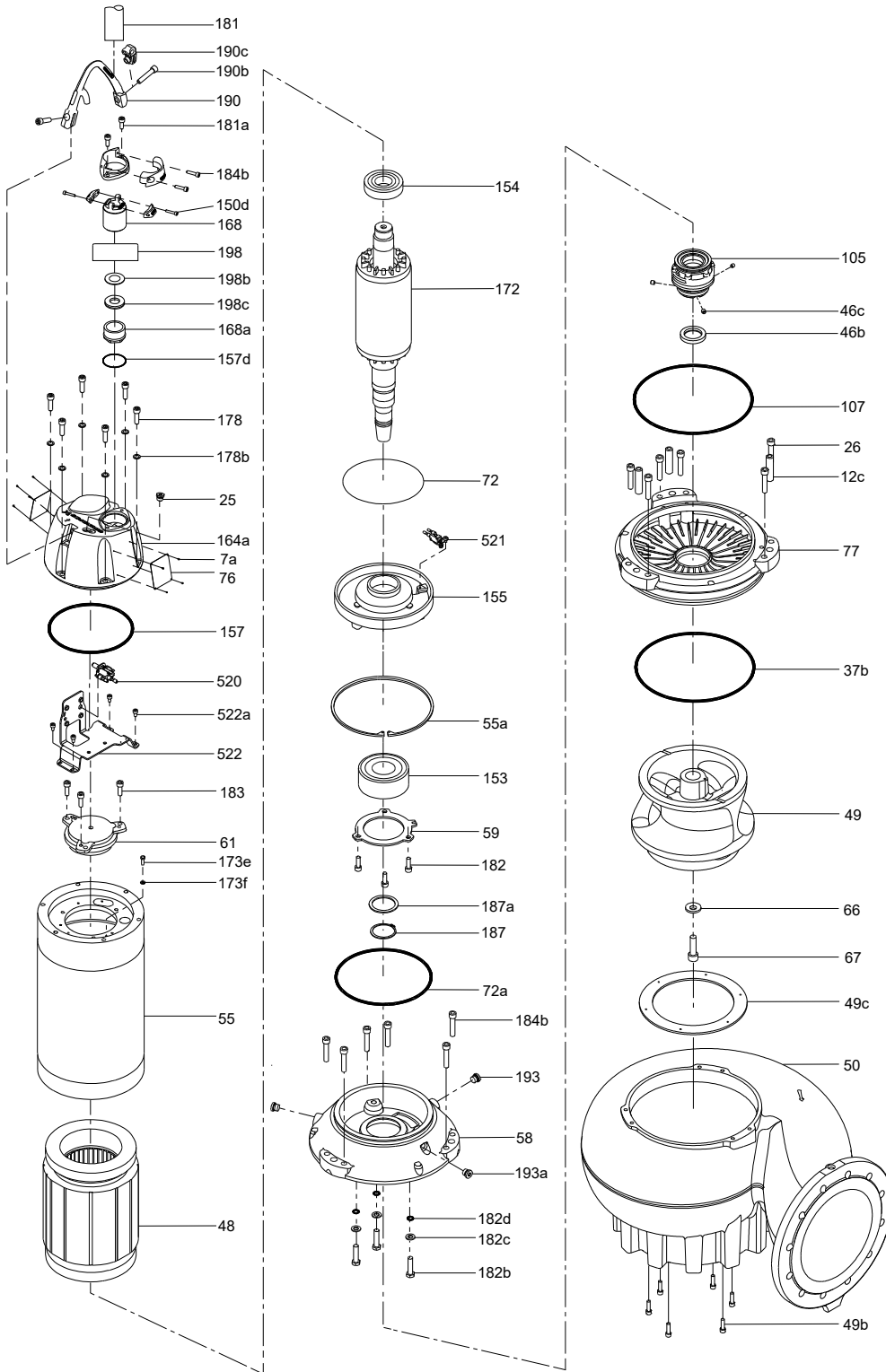
SL2 Ex pumps, 6 poles
