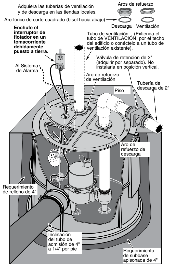
Figura 1 – Instalación típica
